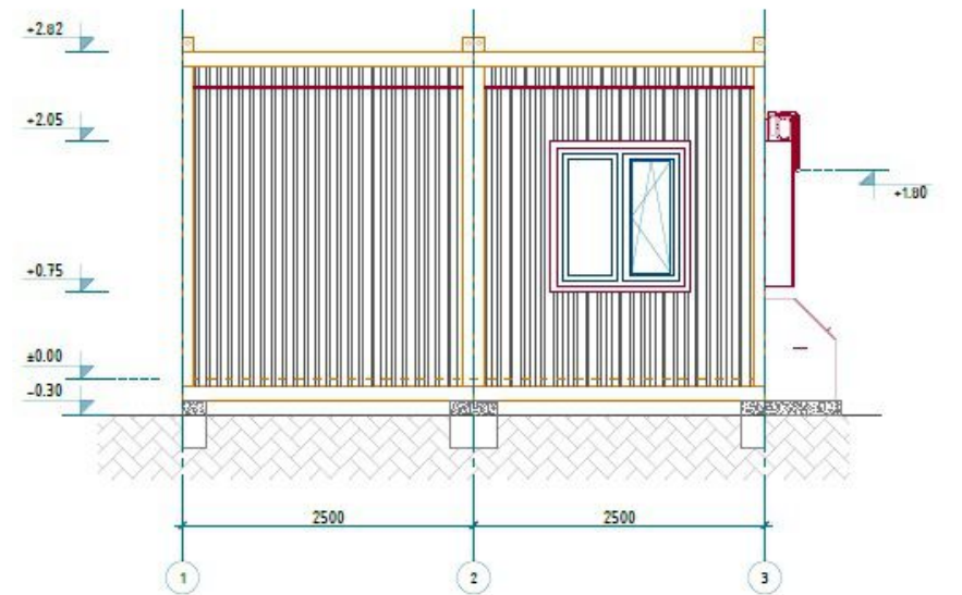
Фасад 1 - 3 М 1:50
