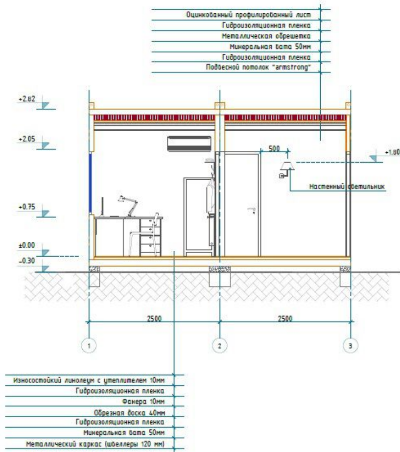
Разрез 1 - 1 М 1:50
