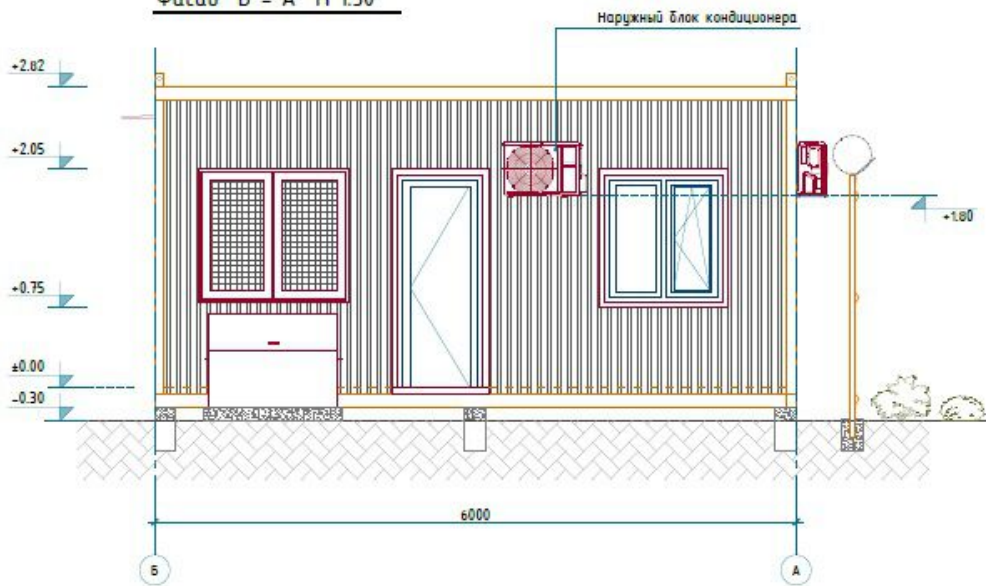
Фасад Б - А М 1:50
