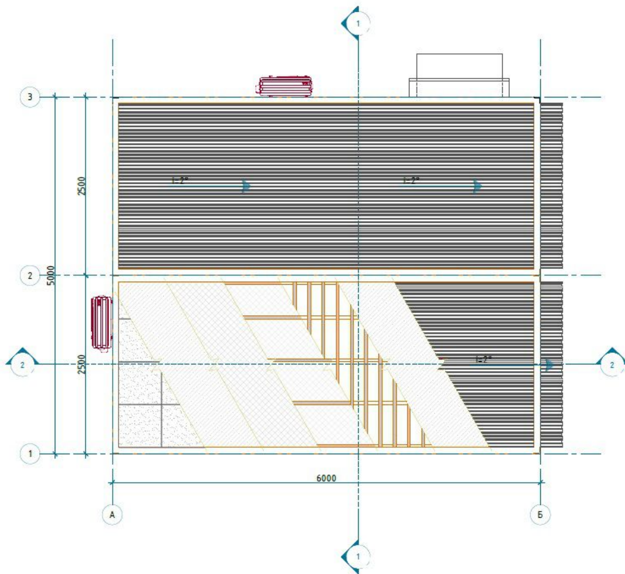
План кровли М 1:50
