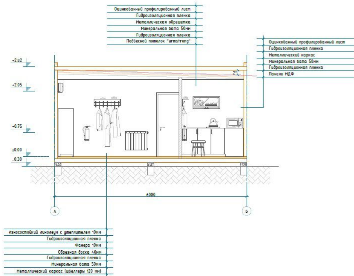
Разрез 2 - 2 М 1:50
