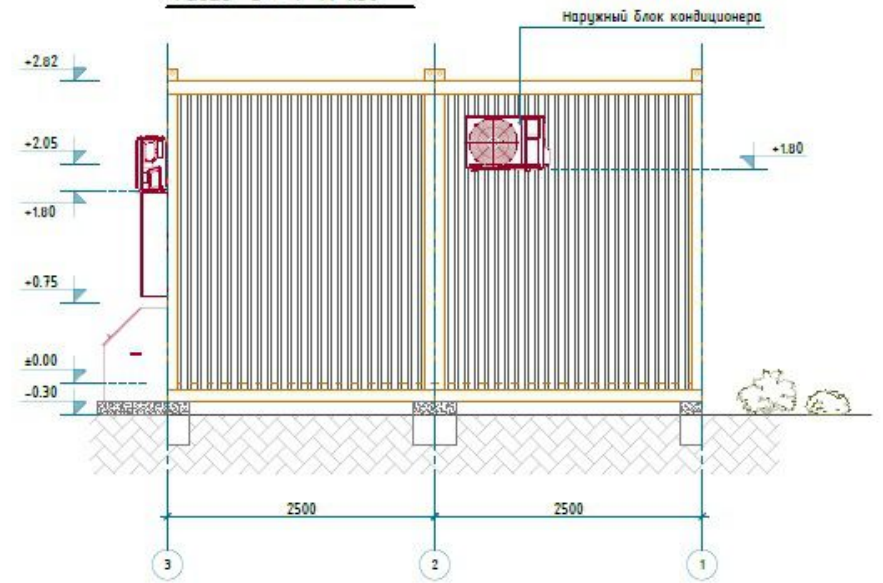
Фасад 3 - 1 М 1:50
