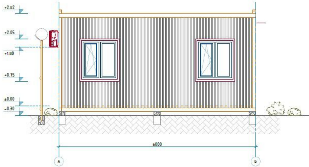
Фасад А - Б М 1:50
