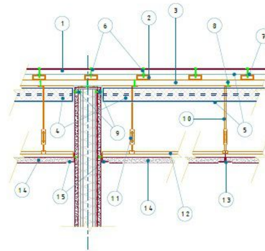
Маркировка деталей узла
