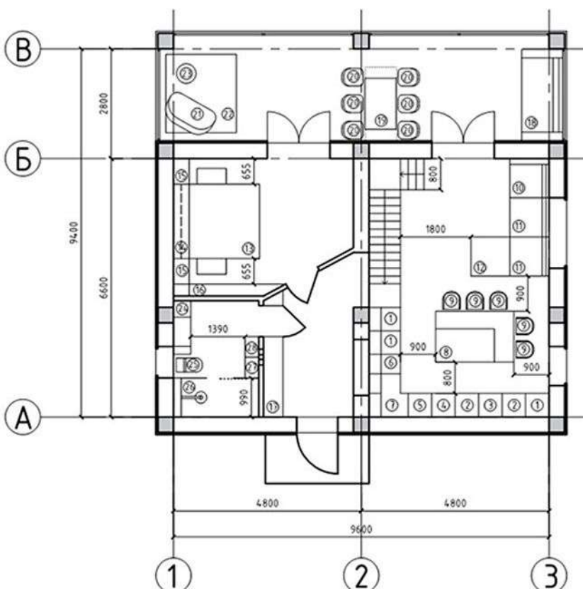
План расстановки мебели первого этажа
