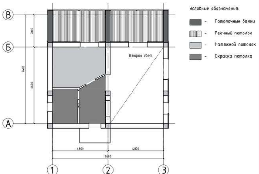
План потолка первого этажа
