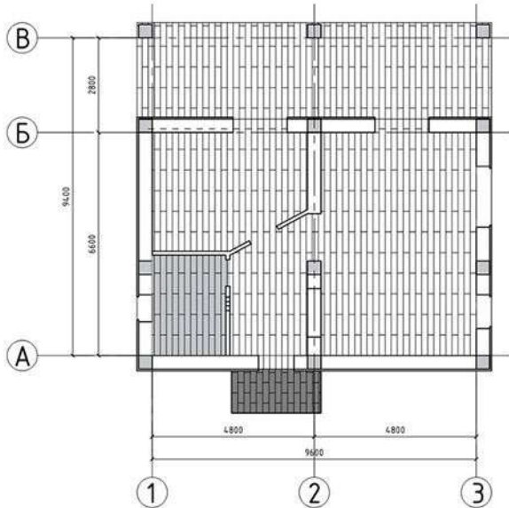
План пола первого этажа
