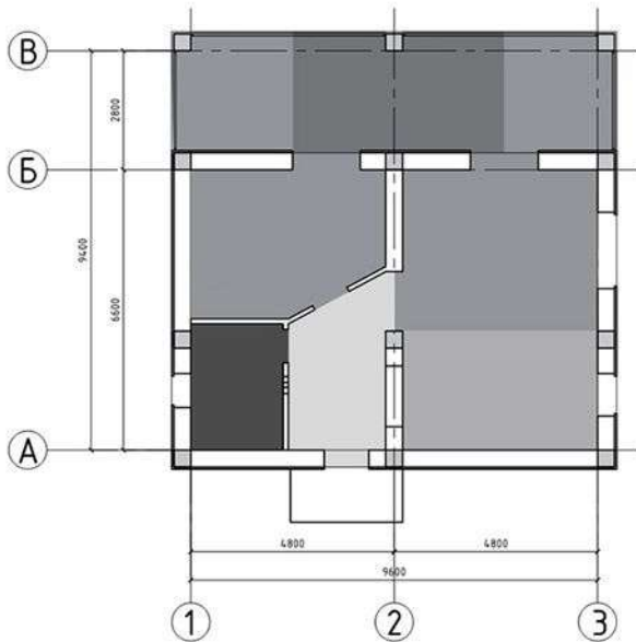
План пола первого этажа
