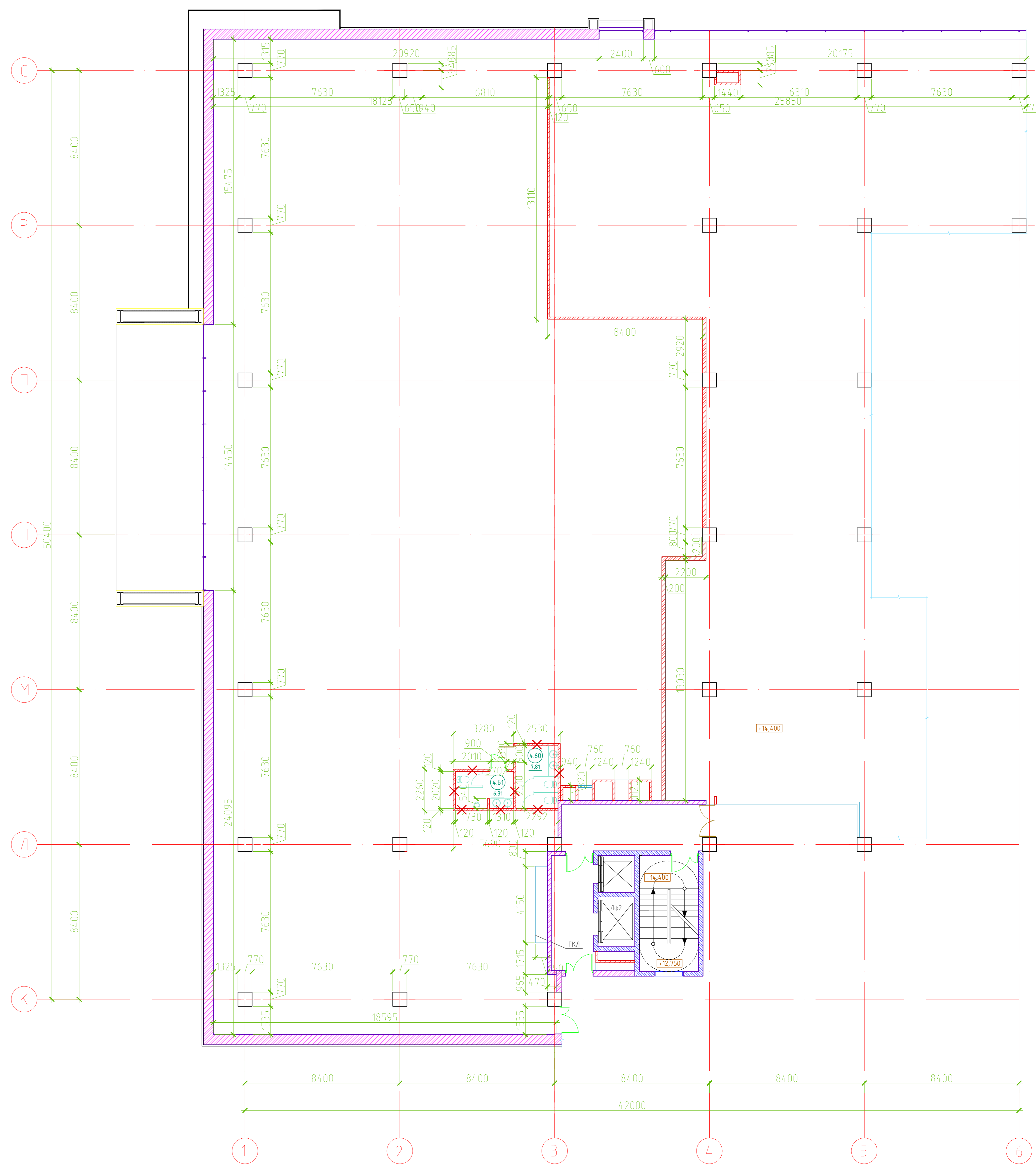
План демонтажа
