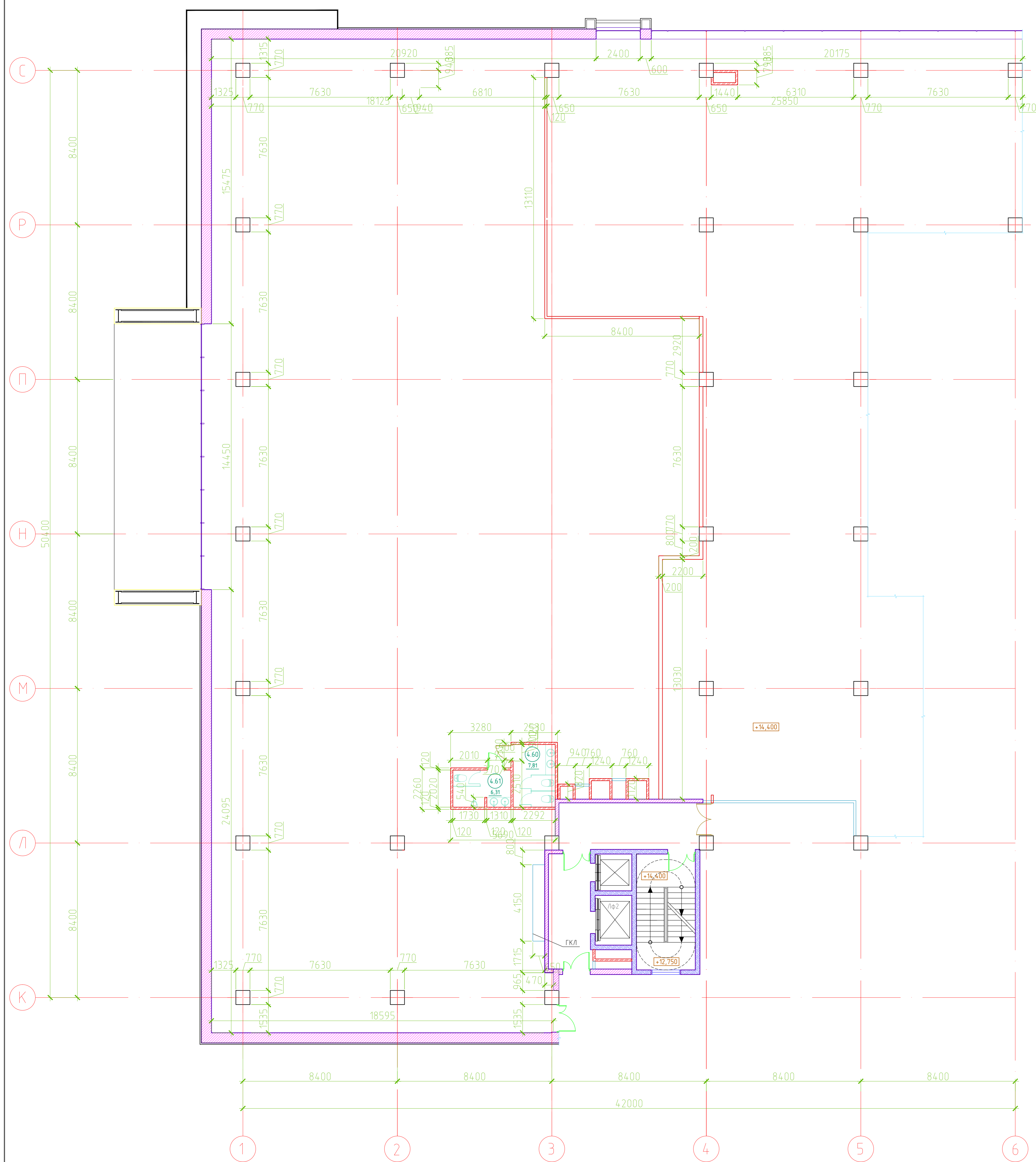
Обмерочный чертеж
