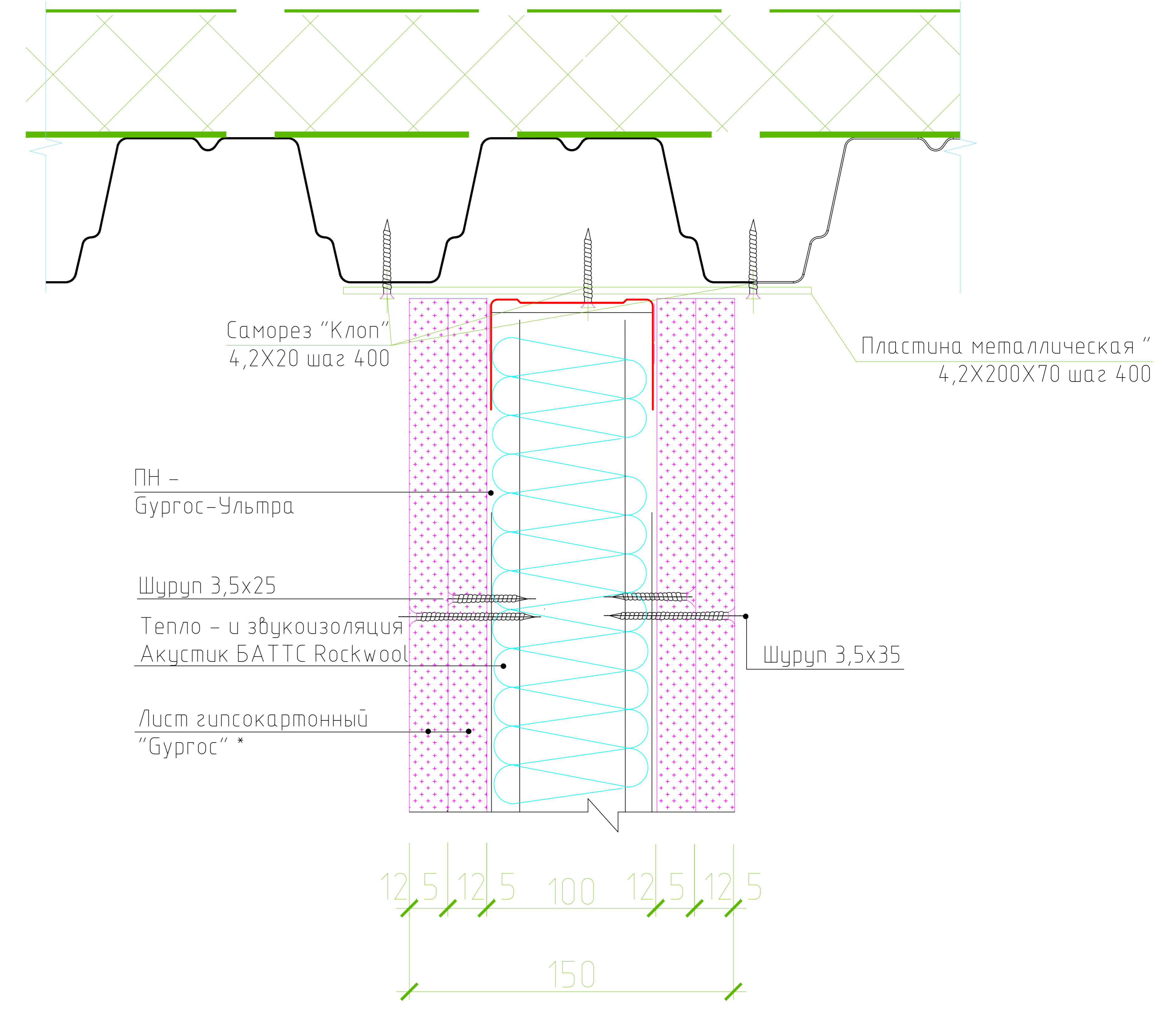
Верхний узел крепления перегородок из ГКЛ (ГКЛВ) к конструкции кровли
