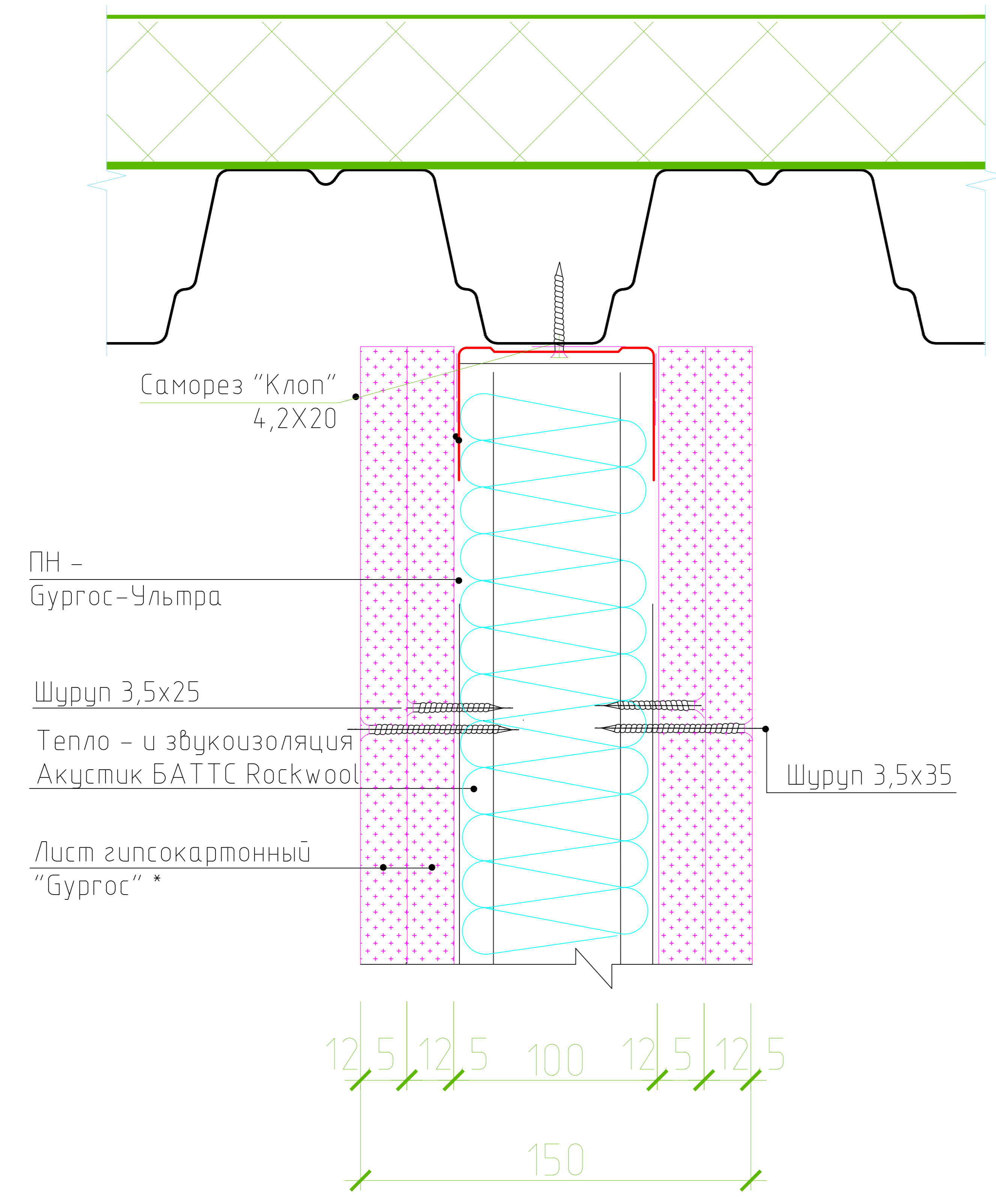
Верхний узел крепления перегородок из ГКЛ (ГКЛВ) к конструкции кровли
